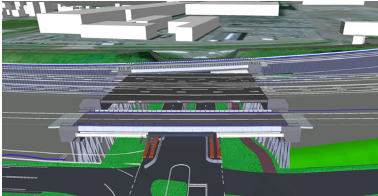
Afbeelding 1 Nieuwe viaducten over Trentweg met tijdelijke ondersteuning
