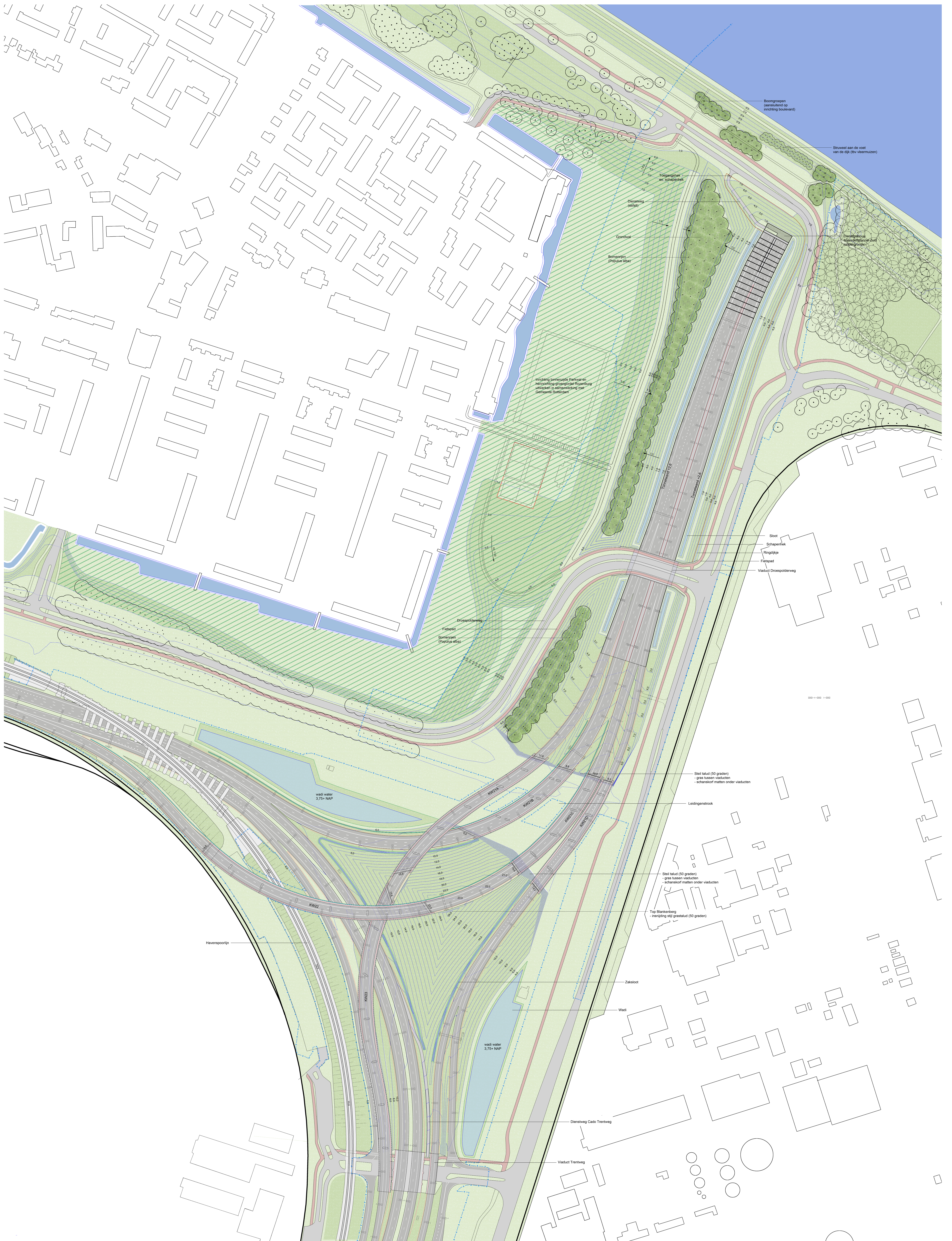
Landschappelijke inpassing Blankenbergverbinding Zuid (schaal 1:1500)
